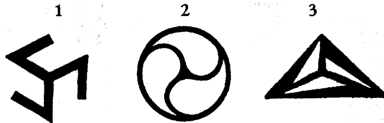
Трискель, трехветвевая свастика: 1 — северный вариант; 2 — кельтский вариант; 3 — «Глаз Дракона»
