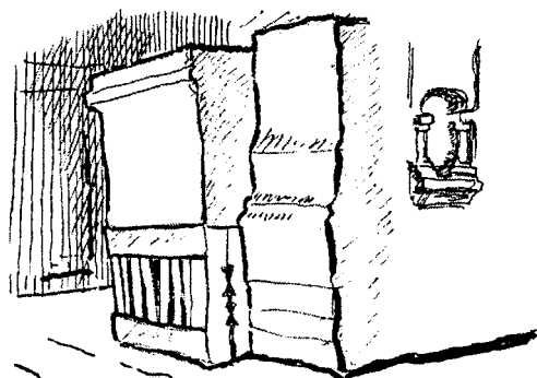
Рис. 31. Печь с курятником в подпечье. Каргопол
