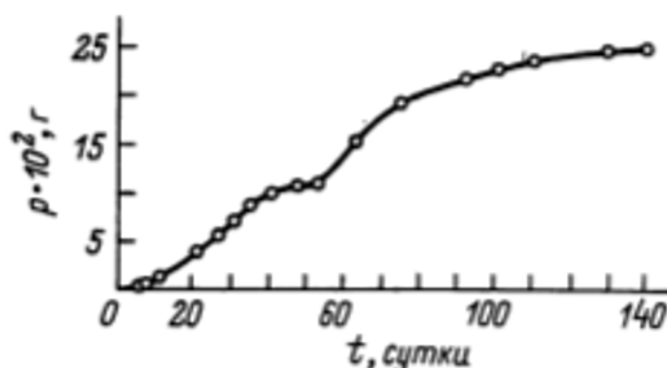
Рис. 6. Кривая зависимости крупности зерен порошка сегнетовой соли от времени.
