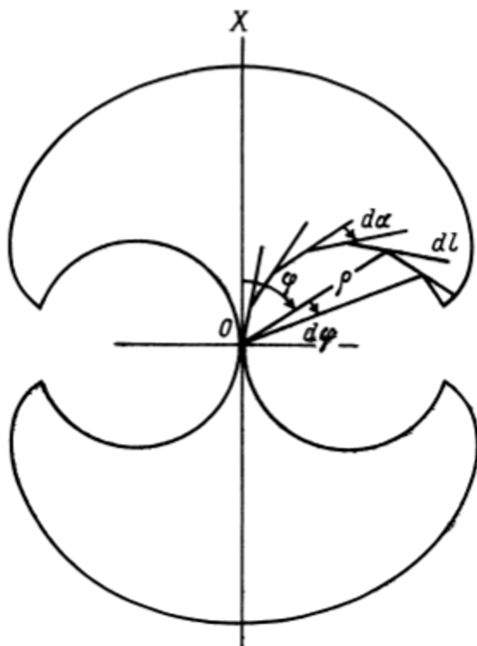
Рис. 10. Пояснение закона образования двулистника с круглыми «глазками».
