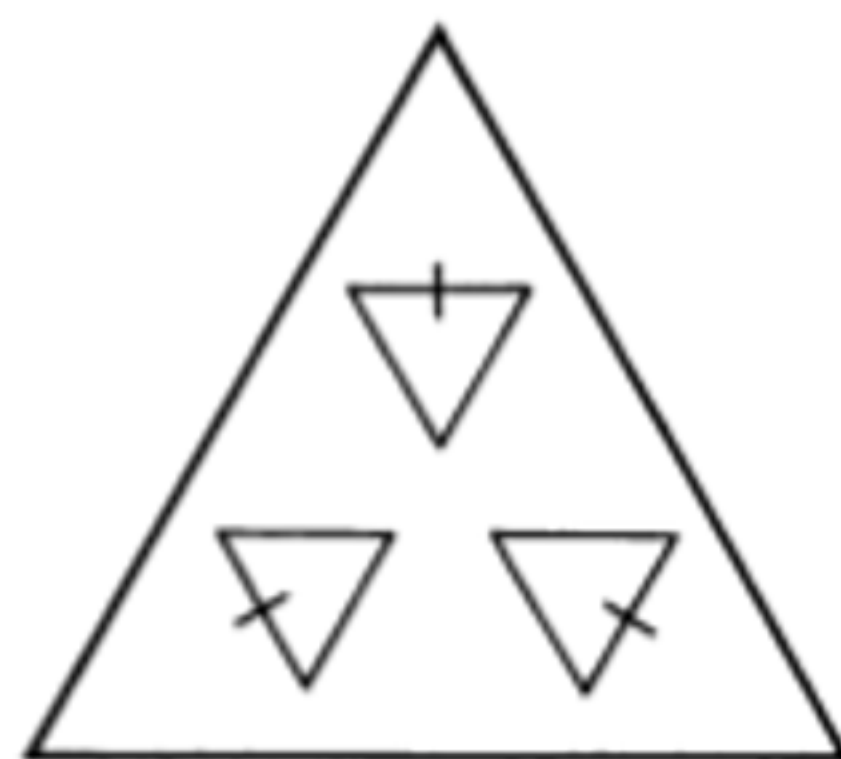
Рис. 5. Положение грани октаэдра на грани октаэдра, приводящее к двойникам по шпинелевому закону.
